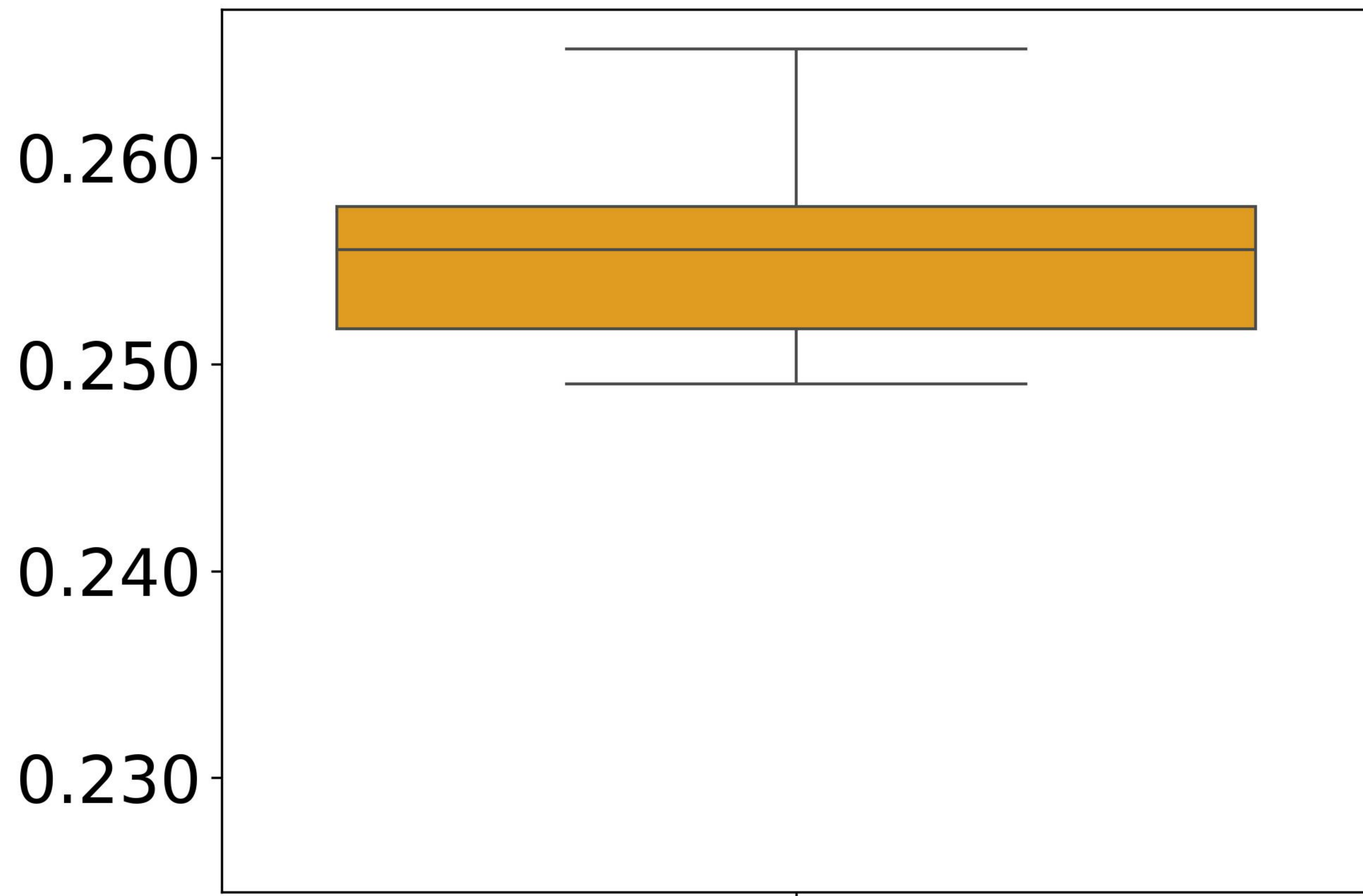
Dense
