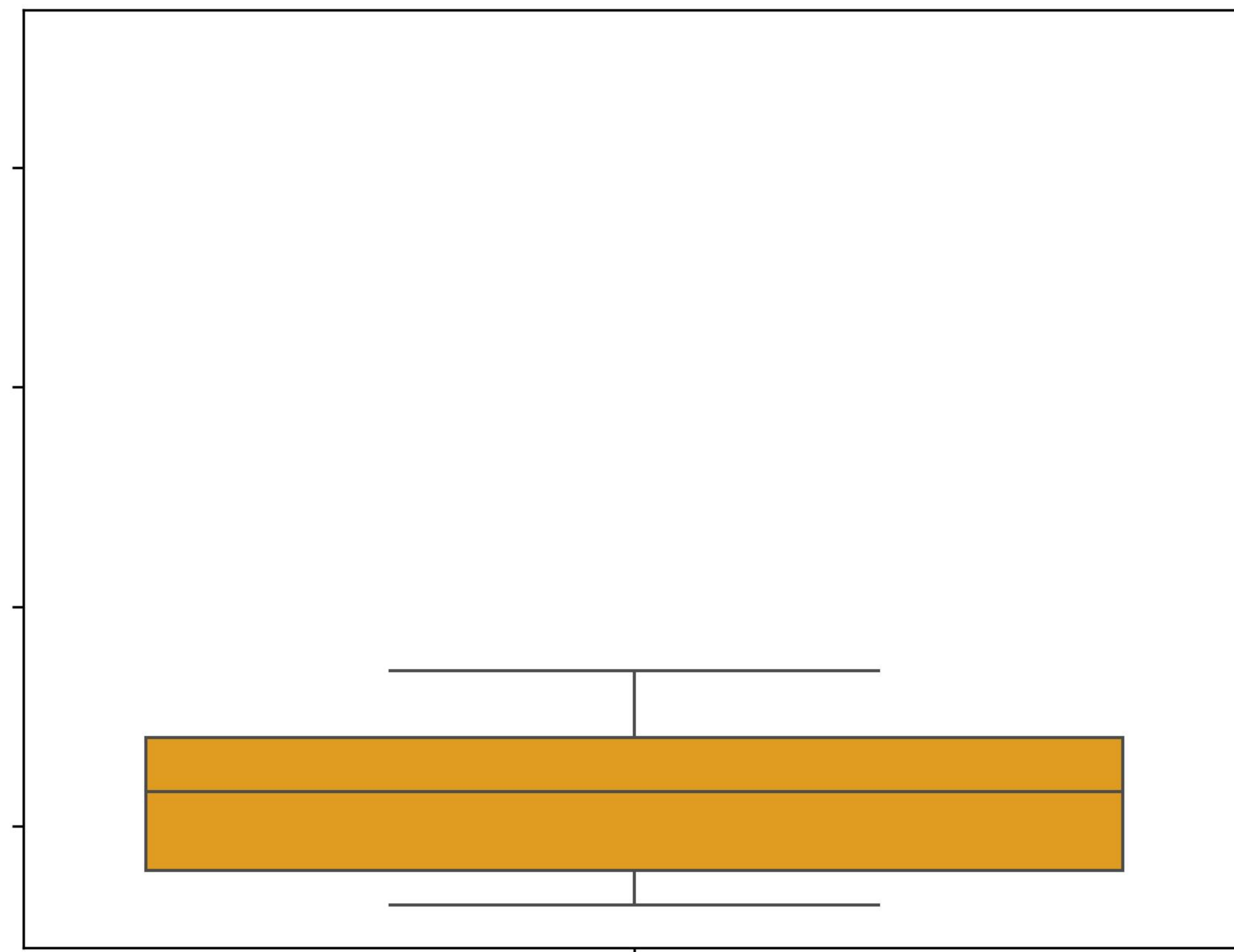
BLSTM
