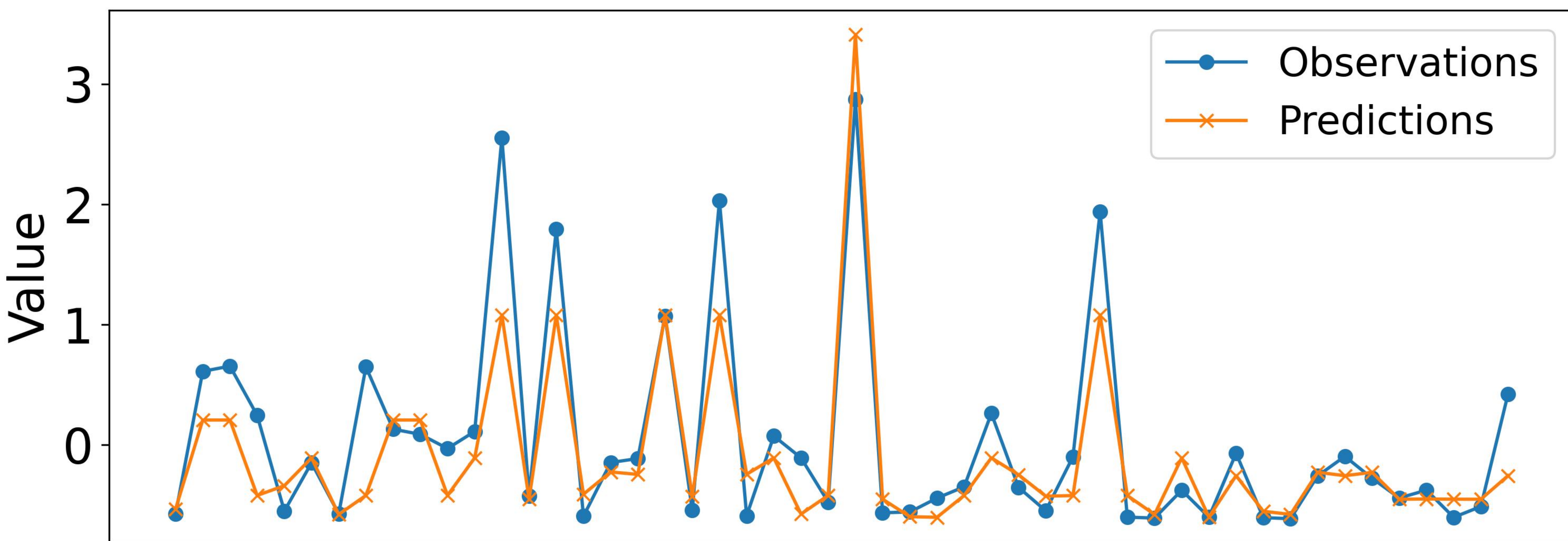
BLSTM
