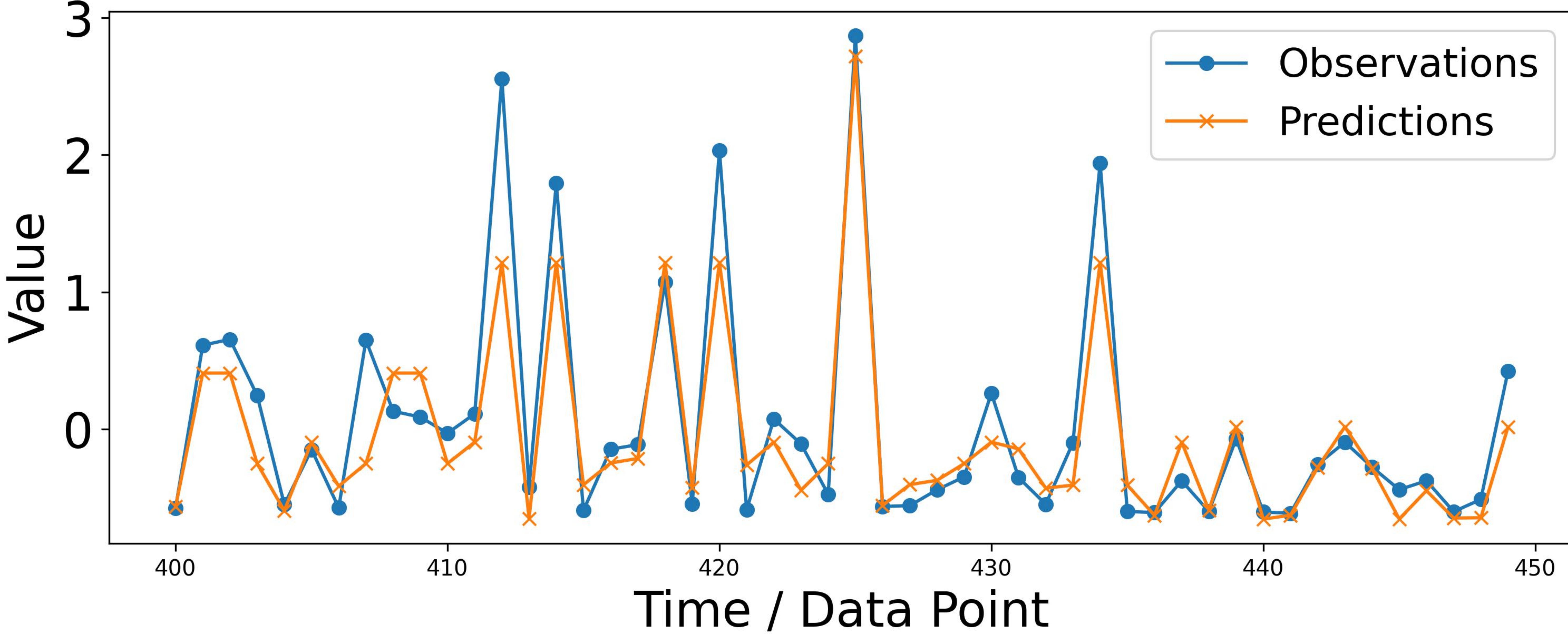
BLSTM
