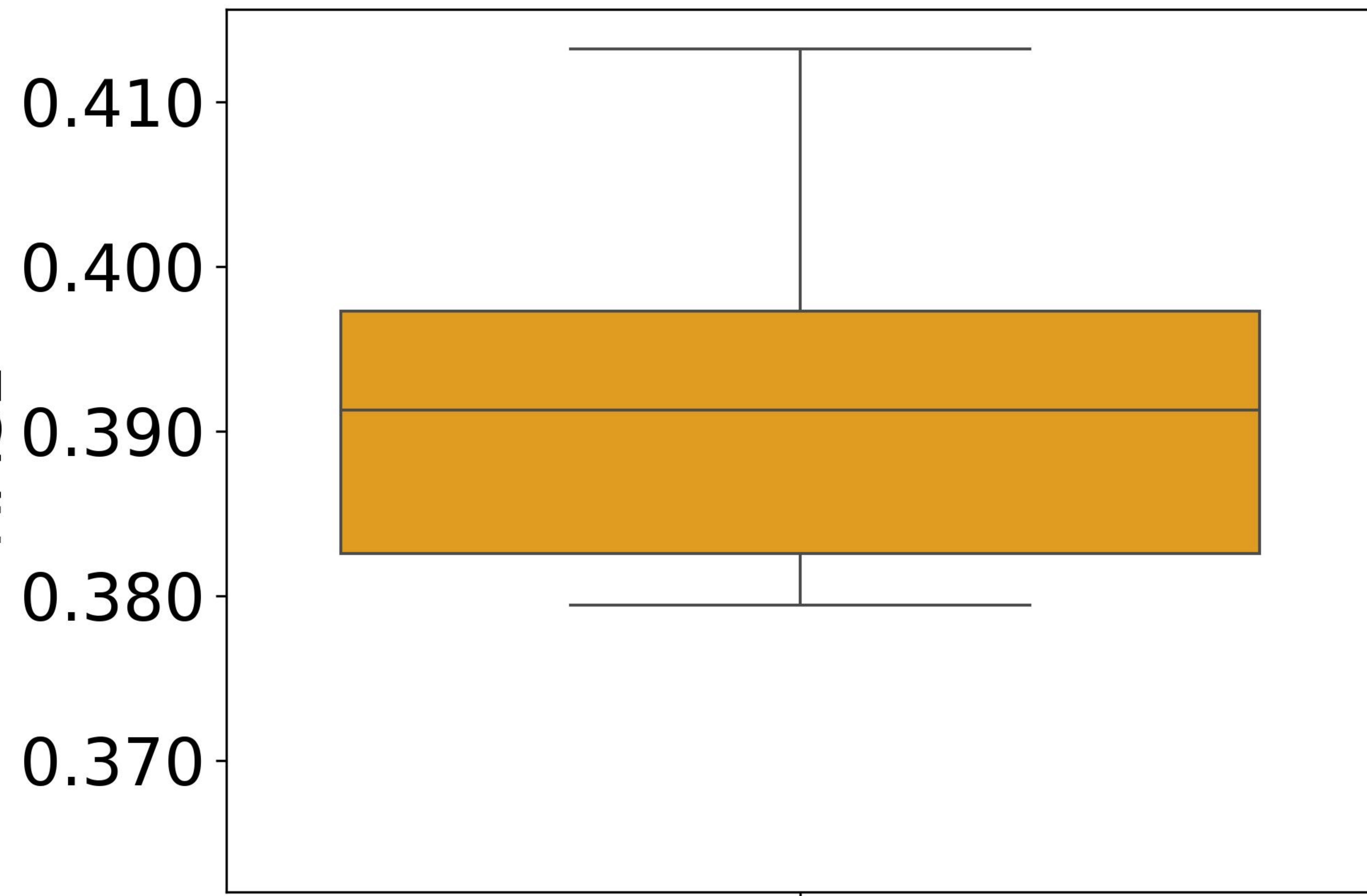
Dense
