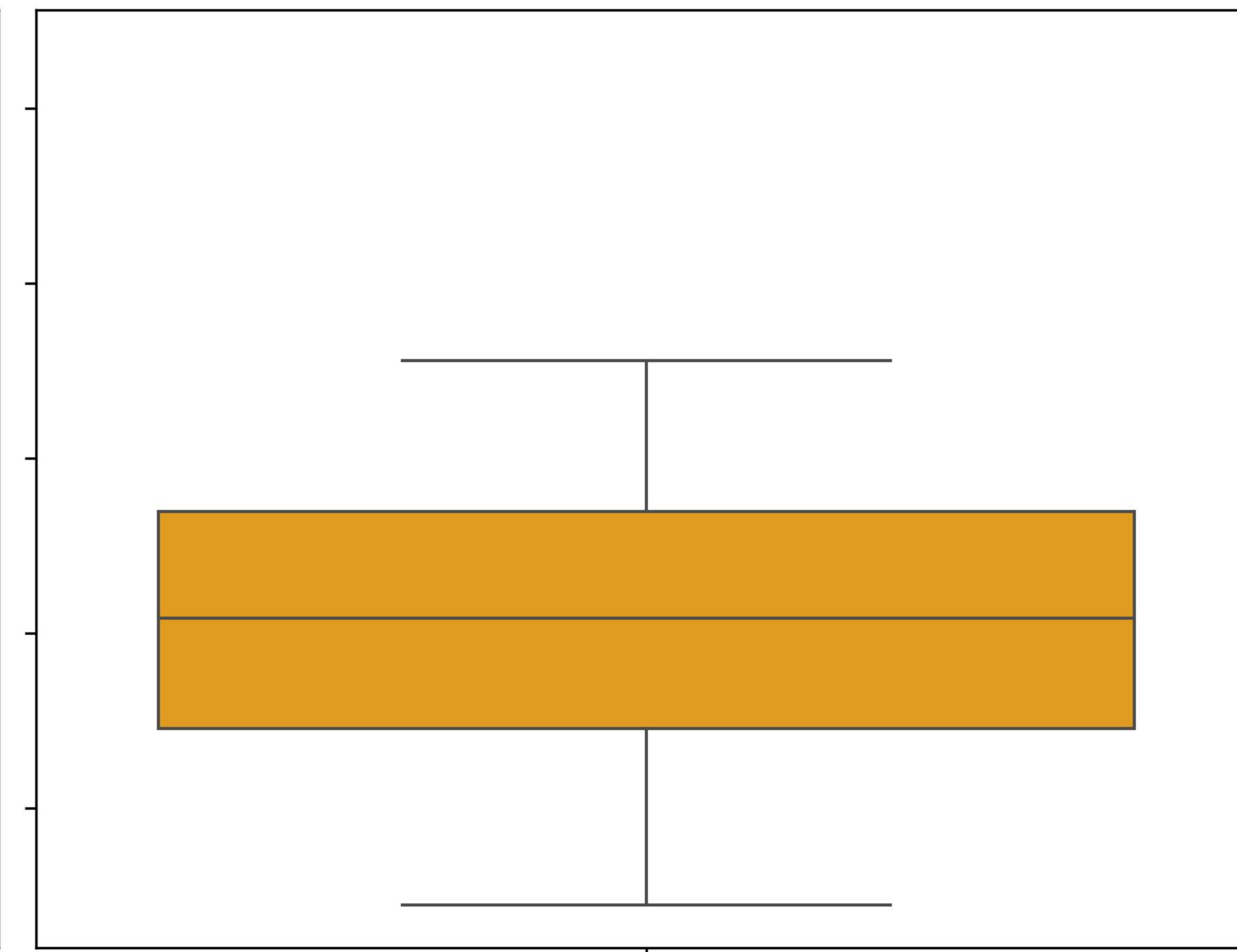
BLSTM
