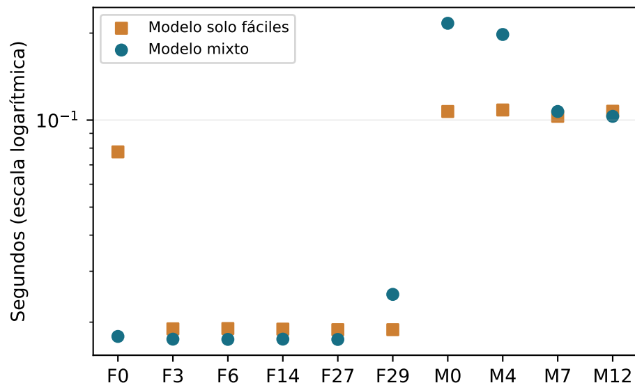
Paso de inferencia en GPU
