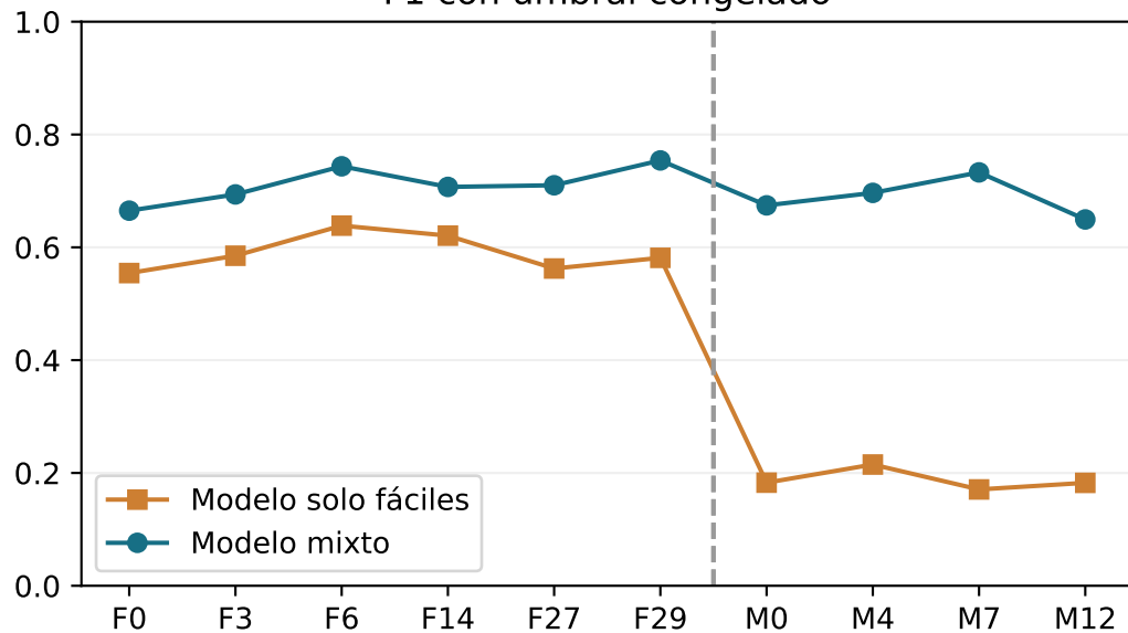
F1 con umbral congelado
