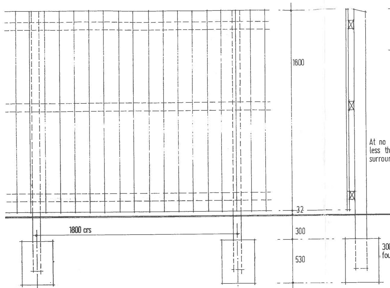
ELEVATION 1:20
