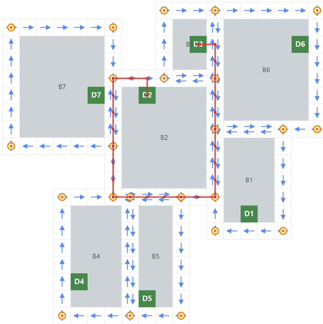
[Fig. 4] move(3, 2, 0, {}) = 26 의 최단경로
