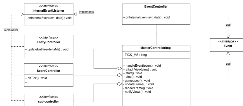
Figura 2.6: Schema UML del MasterController che implementa il GameLoop. sono stati indicati alcuni dei controller principali, quelli non direttamnte specificati sono stereotipati dall interfaccia sub-controller
