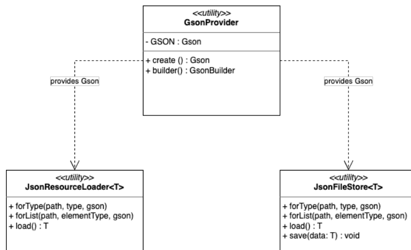
Figura 2.5: Schema UML del sistema per la lettura e scrittura di file JSON
