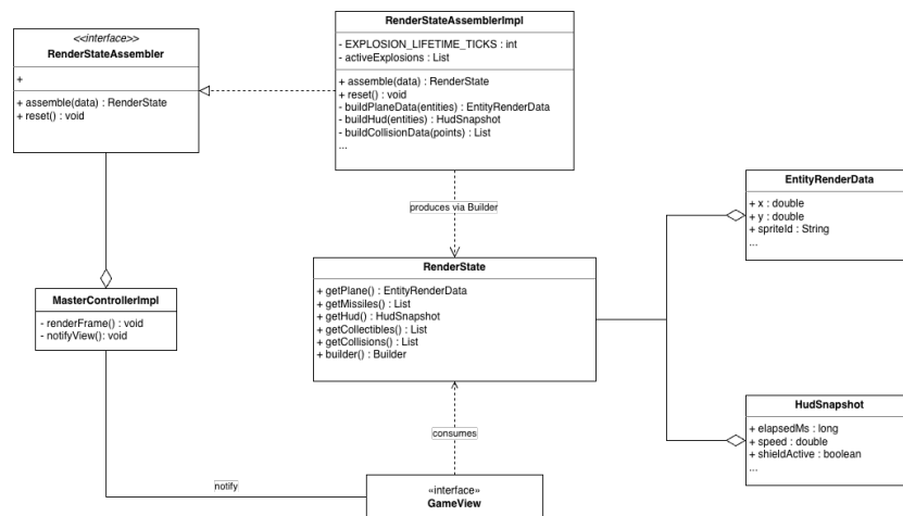
Figura 2.7: Schema UML dell'interazione tra MasterController e RenderStateAssembler per la creazione di RenderState da inviare alla View
