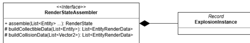
Figura 2.13: Rappresentazione Uml dell'assemblaggio dei render di explosion e collectibles
