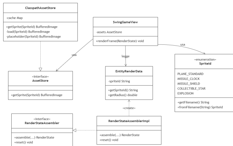
Figura 2.10: Schema UML relativo al asset loader per caricamento di sprite
