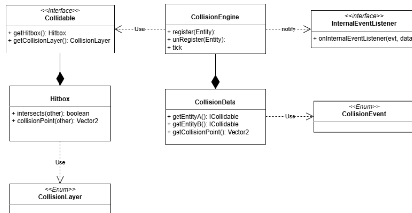
Figura 2.12: Rappresentazione Uml del pattern Observer per gli eventi di collisione
