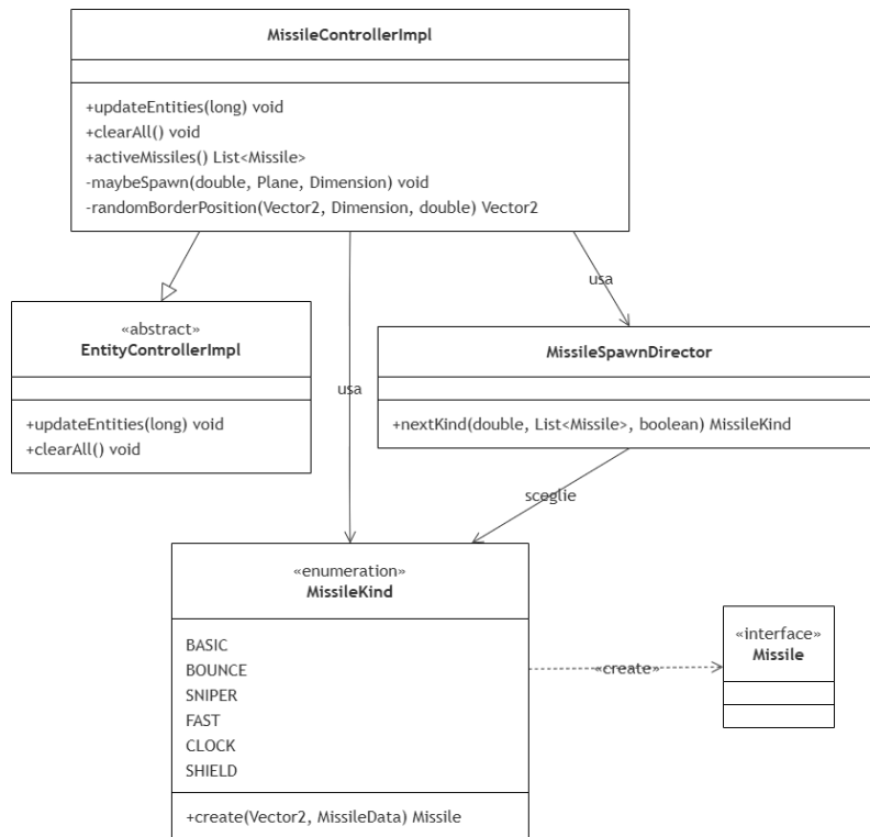
Figura 2.9: Schema UML relativo all'orchestrazione e spawning dei missili
