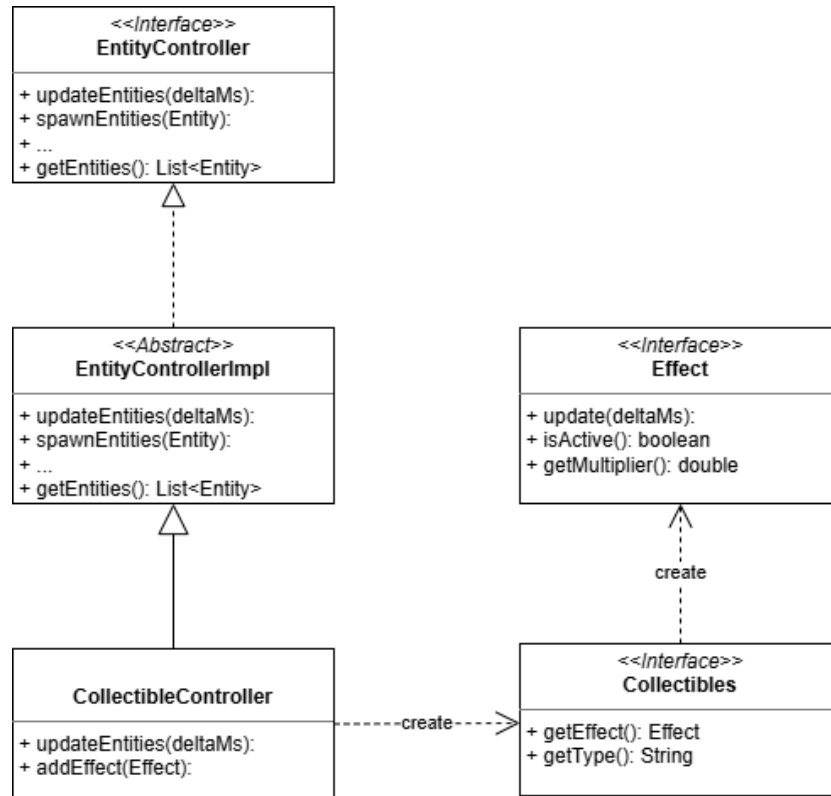
Figura 2.11: Rappresentazione Uml del Pattern Template Method per i controller delle entità e collectibles
