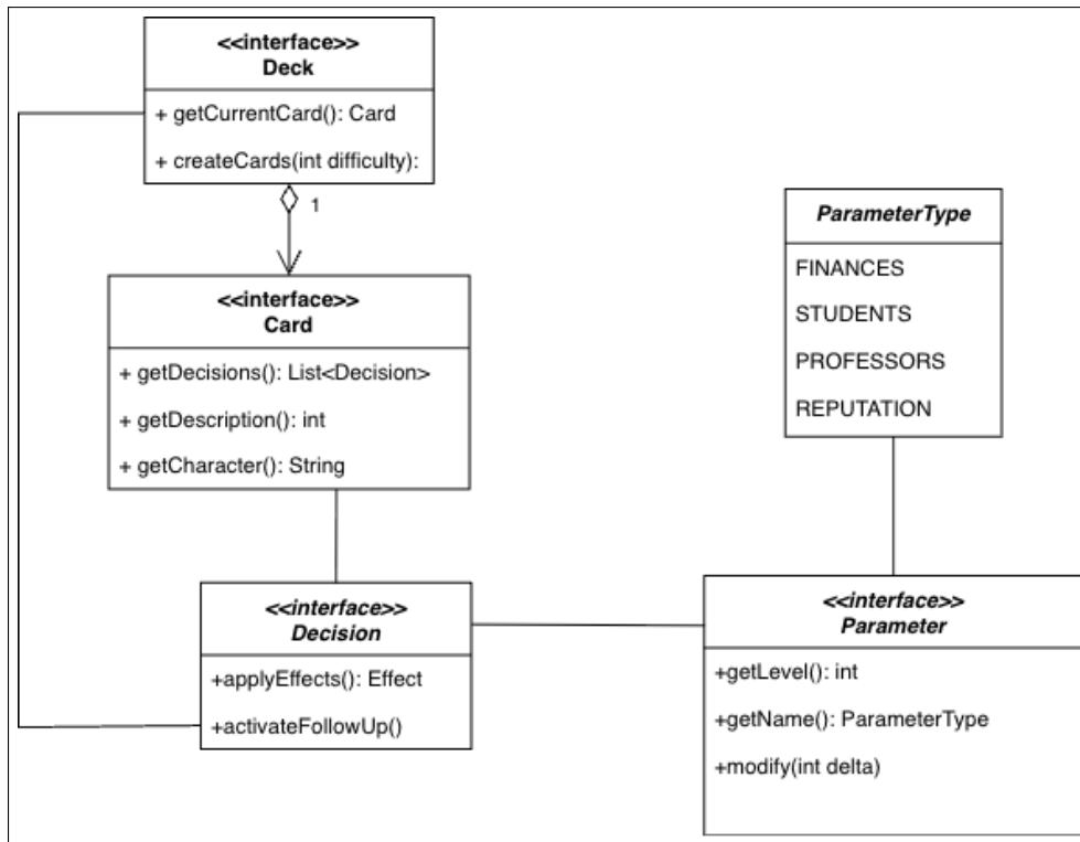
Figura 1.1: Modello del dominio di Aurea Mediocritas: entità, attributi principali e relazioni.
