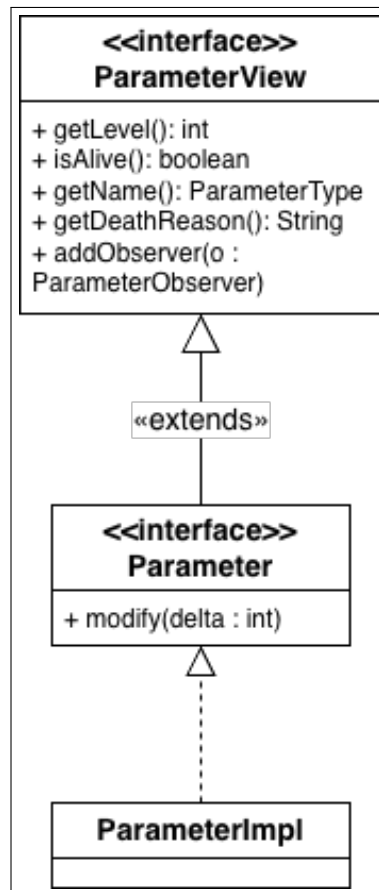
Figura 2.6: Interface Segregation applicata ai parametri di gioco.
