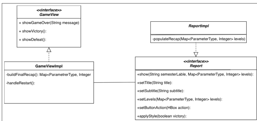
Figura 2.15: Design di ReportImpl come componente riutilizzabile
