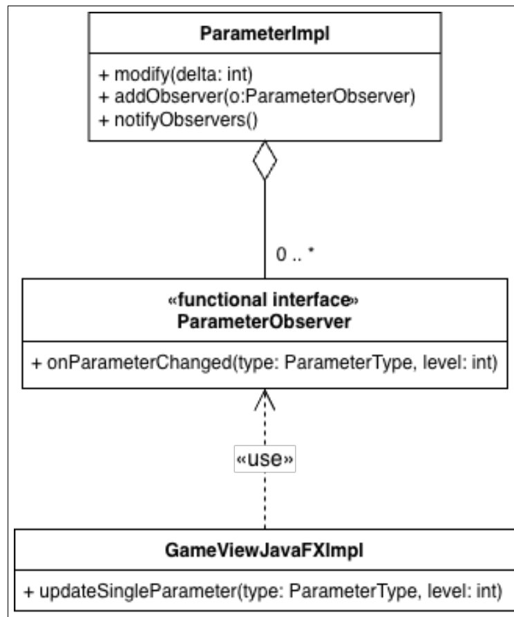
Figura 2.5: Pattern Observer applicato ai parametri di gioco.
