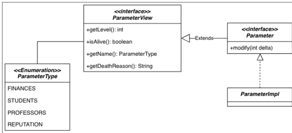
Figura 2.14: Separazione di Parameter e ParameterView
