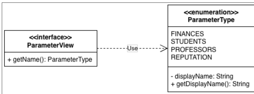
Figura 2.7: Type-Safe Enum con comportamento applicato a ParameterType .
