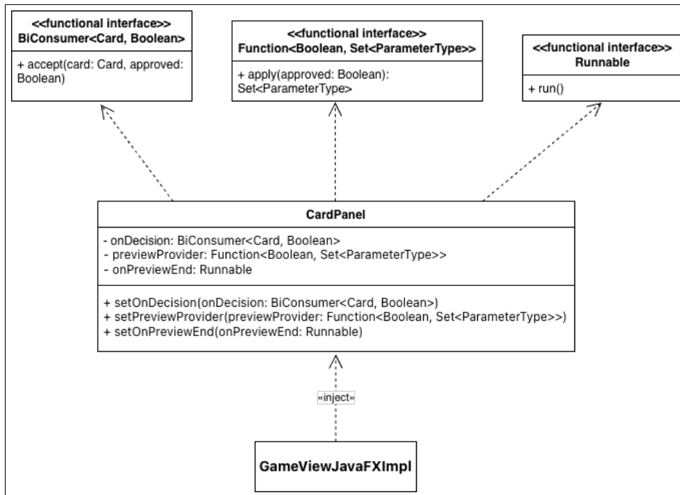
Figura 2.8: Pattern Strategy applicato ai comportamenti di CardPanel.
