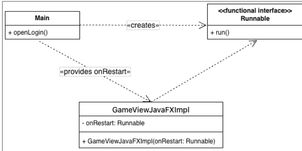
Figura 2.9: Inversion of Control per la gestione del riavvio.
