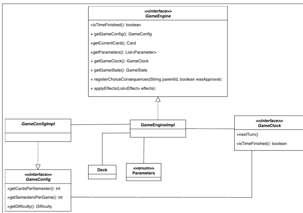
Figura 2.12: Orchestrazione del modello in GameEngineImpl
