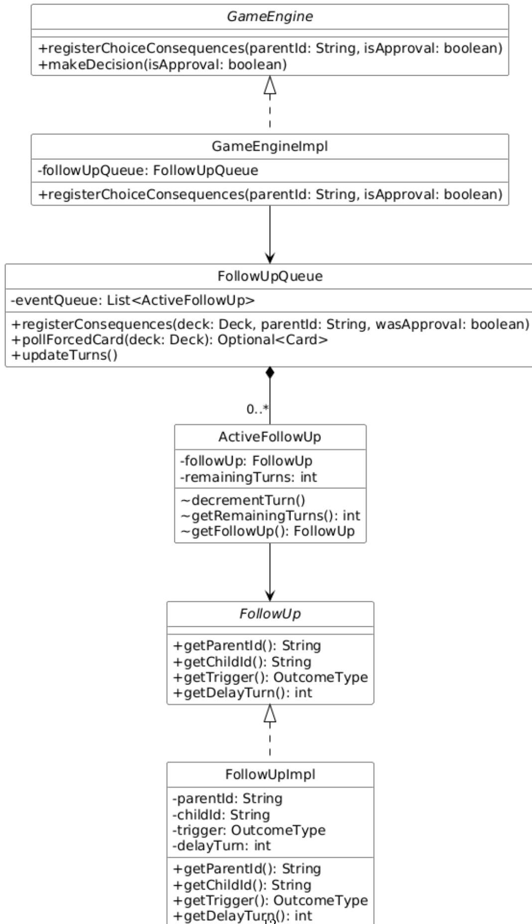
Figura 2.4: Diagramma delle classi UML (Pilastro III): infrastruttura di gestione dei FollowUp. Mostra la composizione FollowUpQueue ◊ ActiveFollowUp (0..*) e la realizzazione
