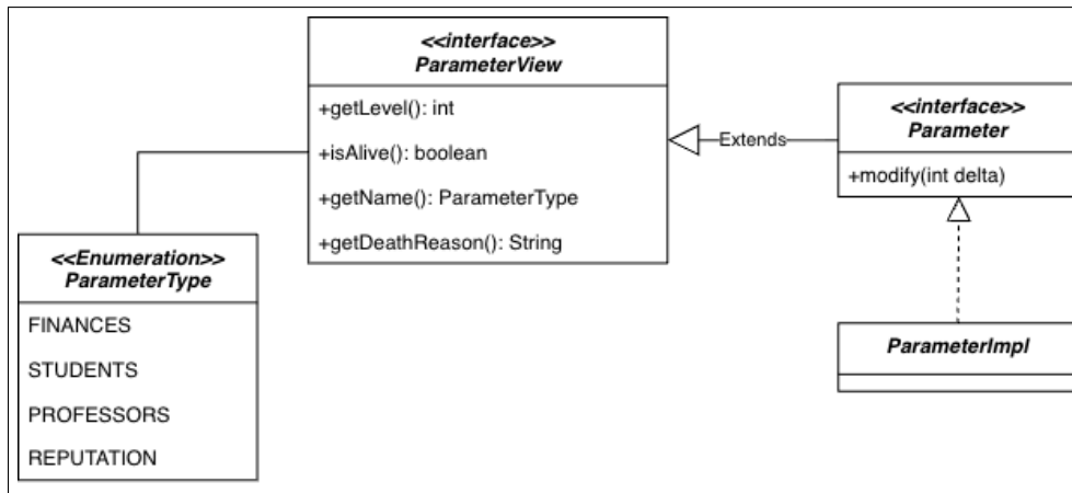
Figura 2.14: Separazione di Parameter e ParameterView
