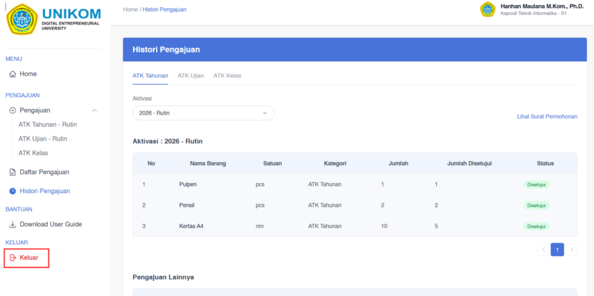
Gambar 1 Halaman Keluar
