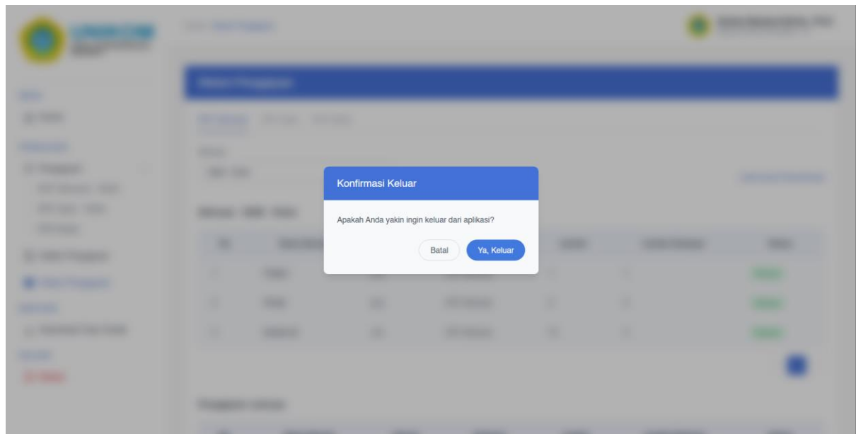
Gambar 2 Halaman Keluar
