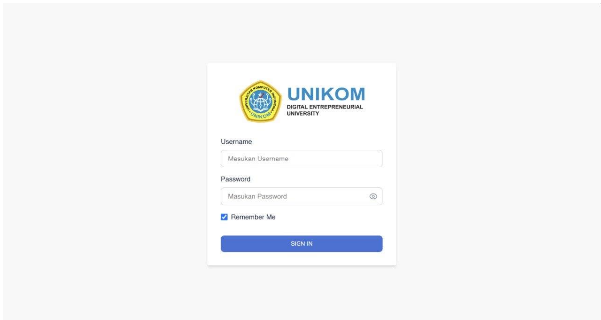
Gambar 1 Halaman Login
