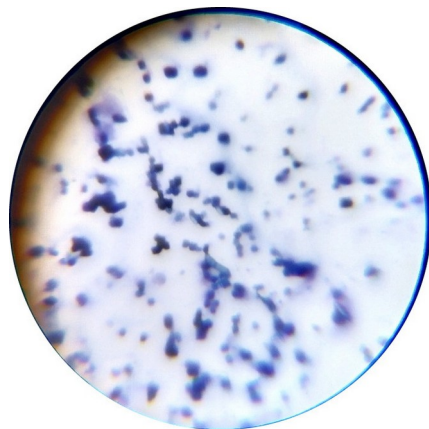
Микроскопия Streptomyces
