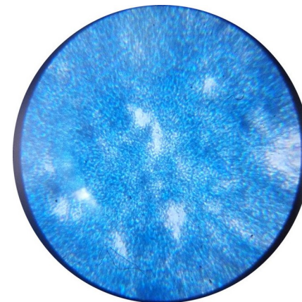
Микроскопия Azotobacter
