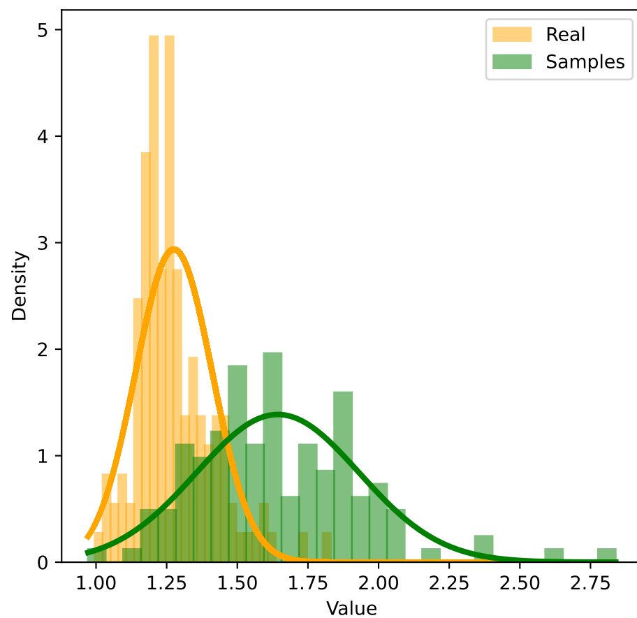
DetectCodeGPT AUC = 0.895285822504516
