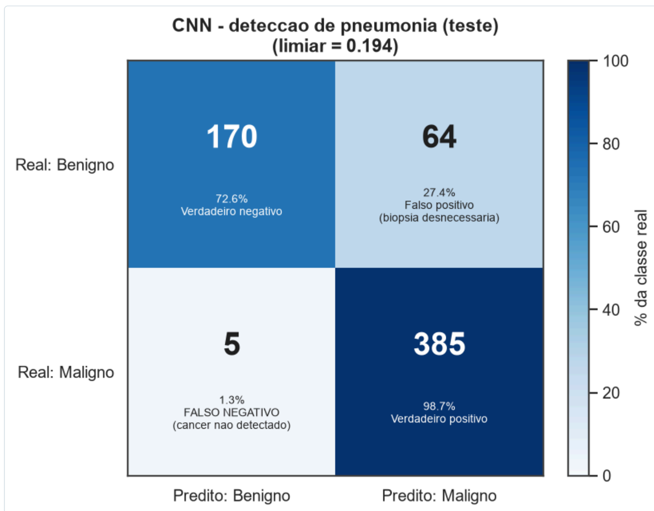
Figura 28. EXTRA: matriz de confusão da CNN no teste. (32_cnn_matriz_confusao.png)
