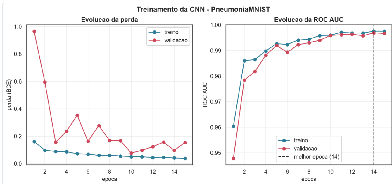
Figura 27. EXTRA: evolução da perda e da ROC AUC ao longo das épocas. (31_cnn_curvas_treino.png)
