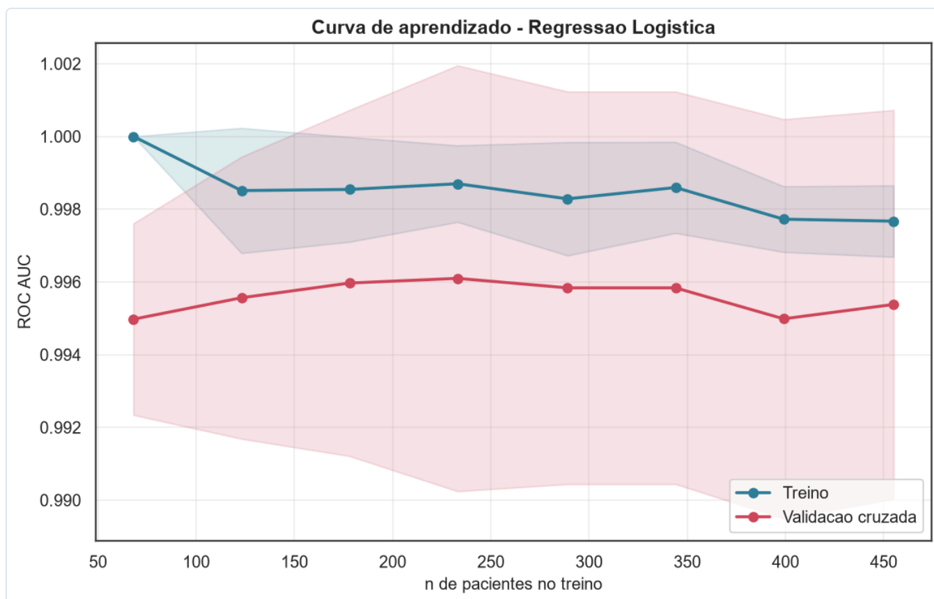
Figura 16. Curva de aprendizado do modelo campeão. (16_curva_aprendizado.png)
