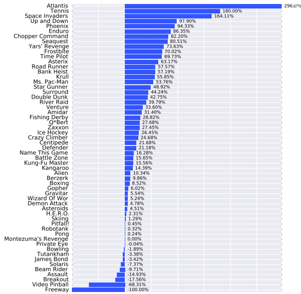
图 4. 决斗架构相对于 van Hasselt 等人的基线单一网络的改进。（2015），使用等式（10）中描述的度量。右侧的条形表示决斗网络优于单流网络的程度。
