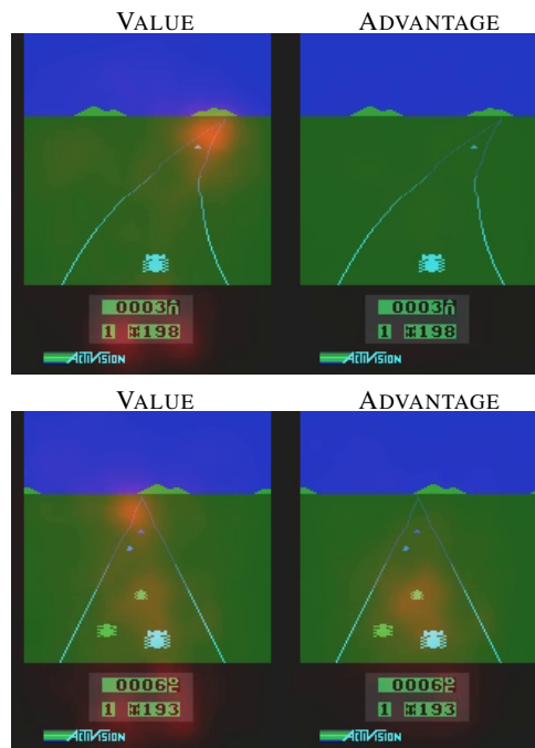
图 2. 查看、参与和驾驶：Atari 游戏 Enduro 上的价值和优势显着性地图（红色叠加），用于训练有素的决斗架构。价值流学会关注道路。优势流学会仅在前方有汽车时才注意，以避免碰撞。
