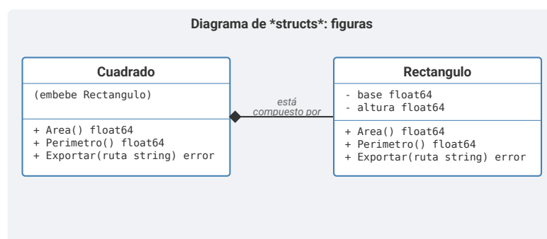
Figura 2.14: Diagrama de structs del ejercicio de figuras geométricas.
