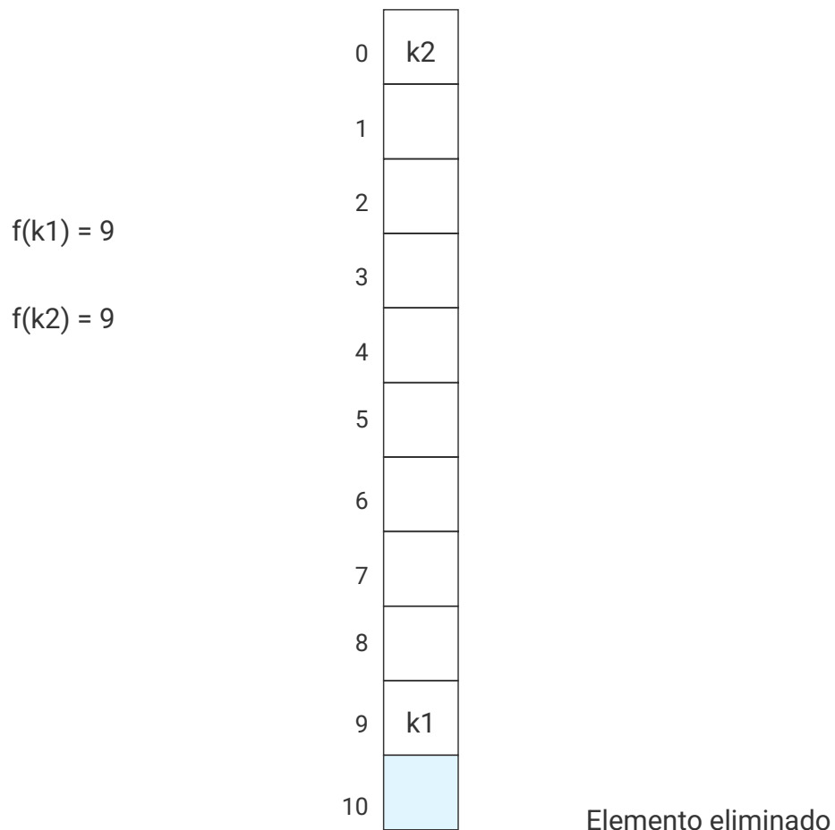
Figura 5.75: Eliminación en una tabla de hash cerrada.
