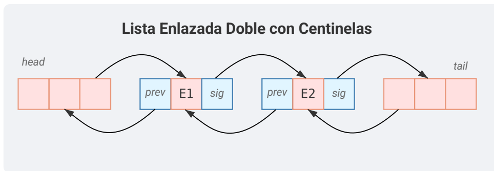
Figura 5.56: Lista Enlazada Doble con Centinelas
