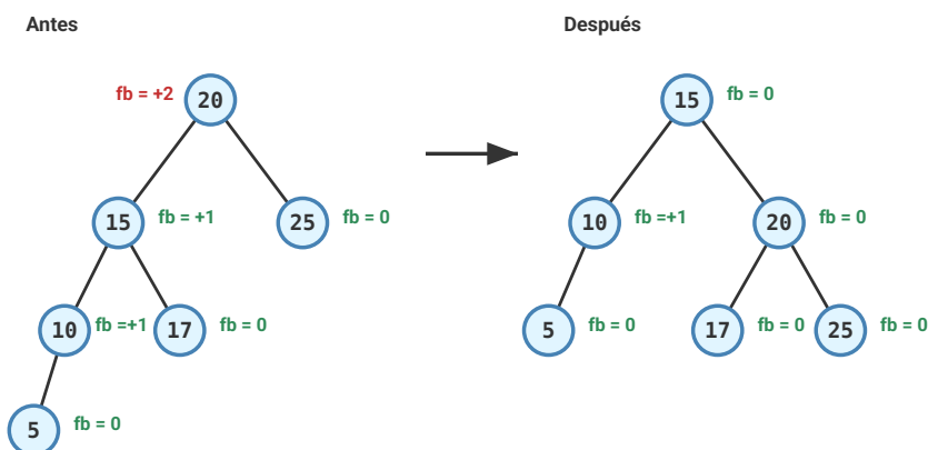
Figura 5.92: Rotación simple a derecha del nodo (20)
