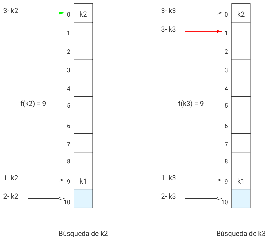
Figura 5.76: Búsqueda en una tabla de hash cerrada.
