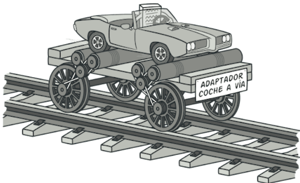
Figura 6.3: Patrón Adapter
