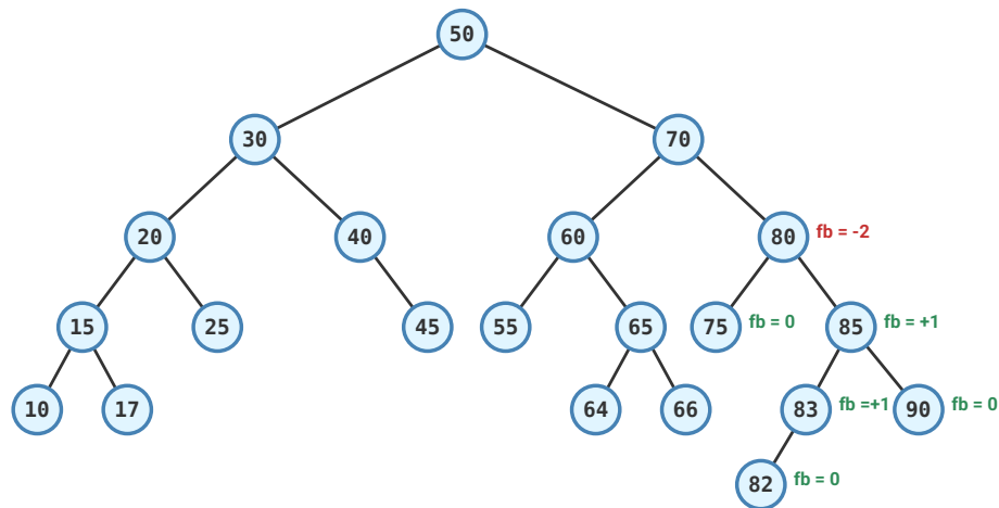
Figura 5.102: Desbalanceo Derecha-Izquierda: fb(80) = -2 , fb(85) = +1
