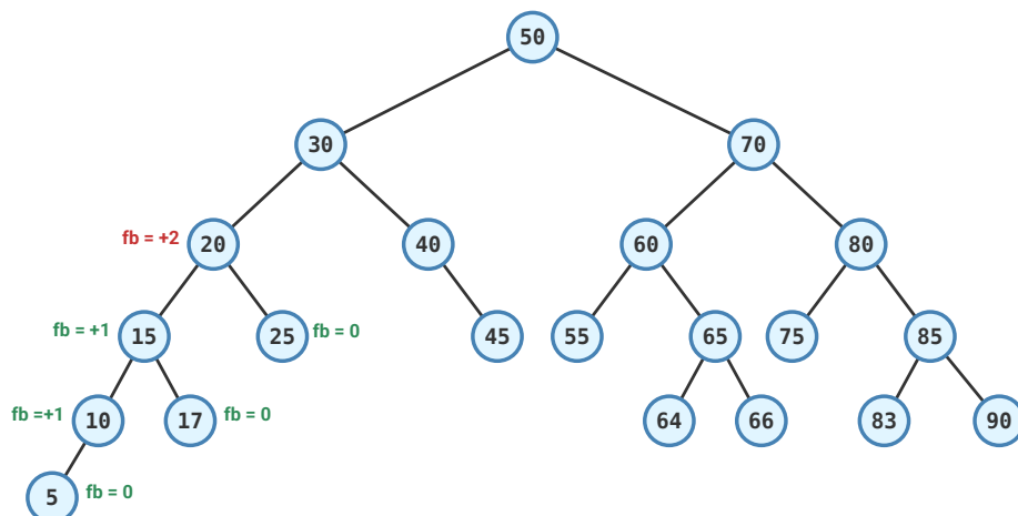
Figura 5.91: Desbalanceo Izquierda-Izquierda: fb(20) = +2
