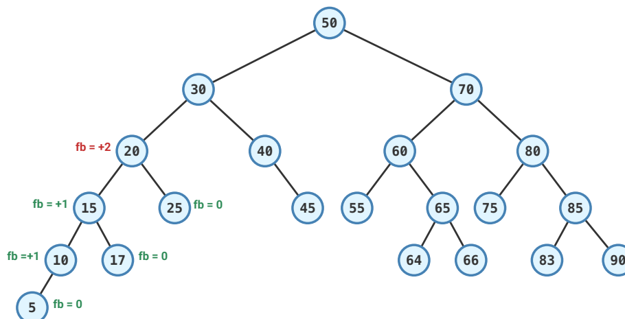
Figura 3.89: Desbalanceo Izquierda-Izquierda: fb(20) = +2
