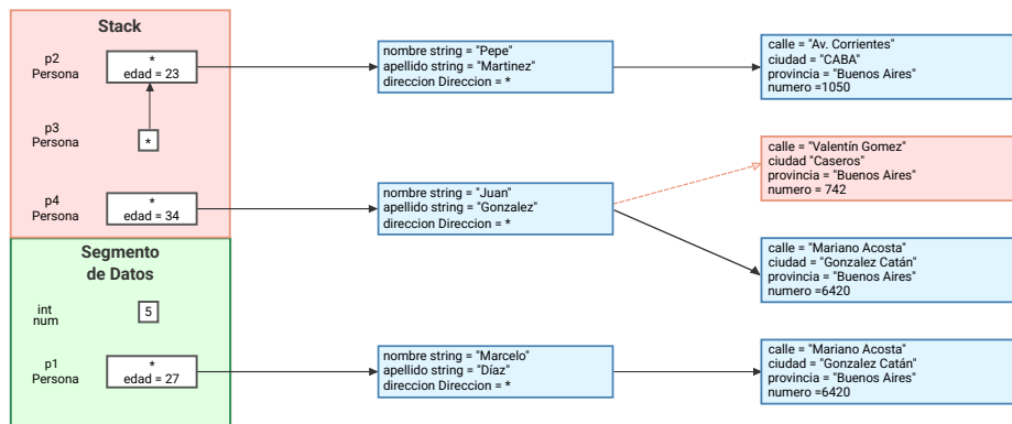
Figura 1.2: Mapa de Memoria
