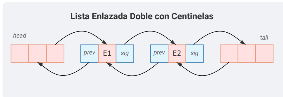
Figura 3.54: Lista Enlazada Doble con Centinelas
