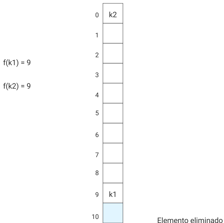
Figura 3.73: Eliminación en una tabla de hash cerrada.
