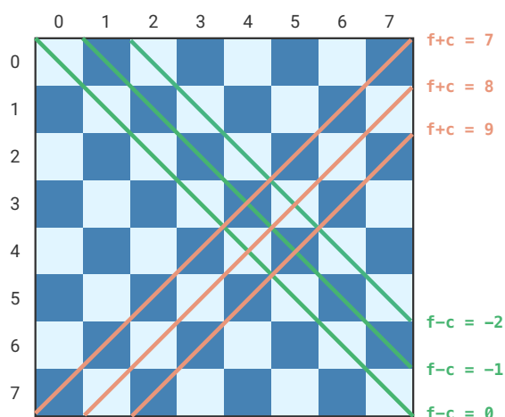
Figura 4.15: Reinas en la misma diagonal
