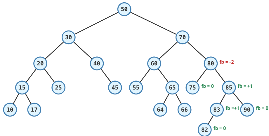
Figura 3.100: Desbalanceo Derecha-Izquierda: fb(80) = -2 , fb(85) = +1
