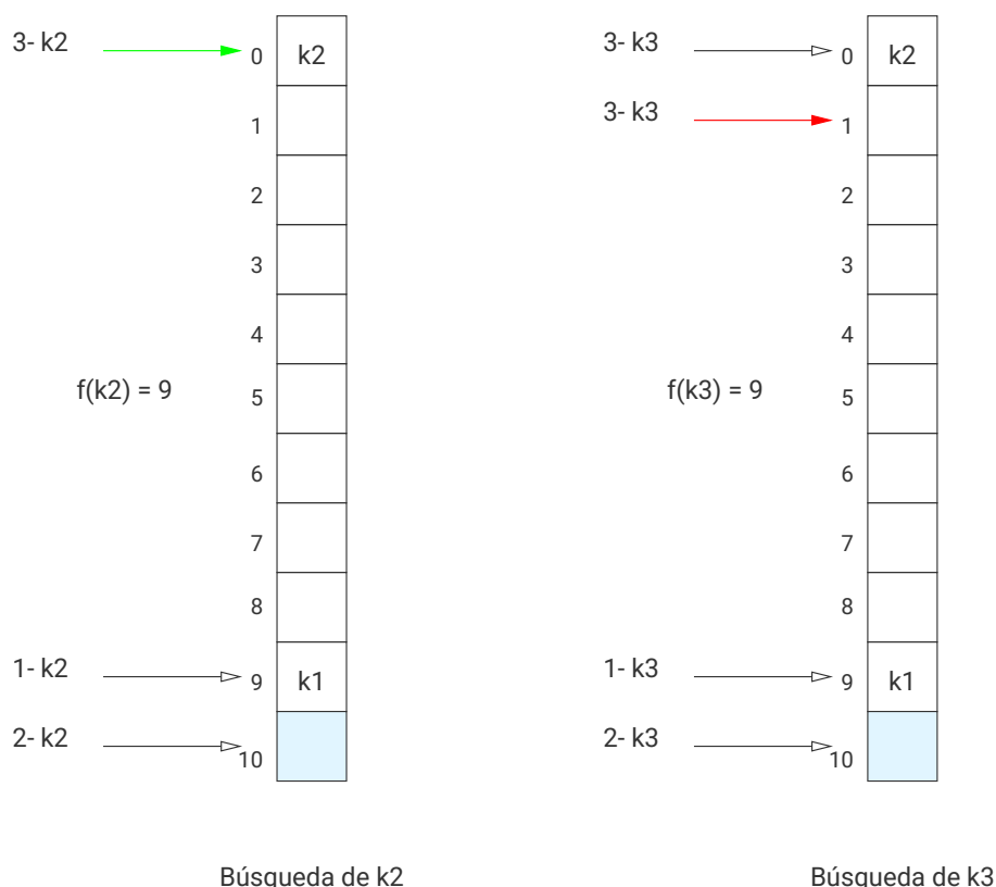
Figura 3.74: Búsqueda en una tabla de hash cerrada.
