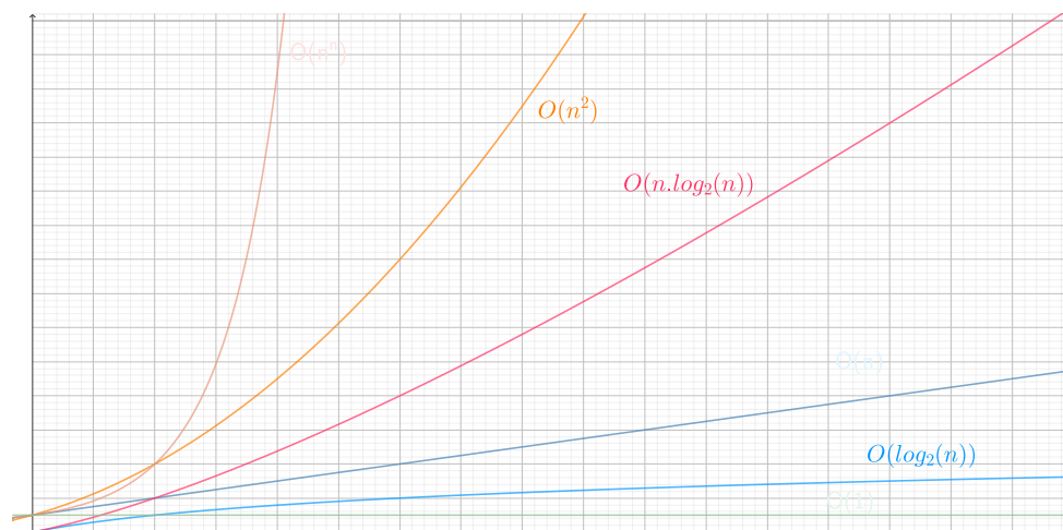
Figura 1.4: Comparación de tasas de crecimiento
