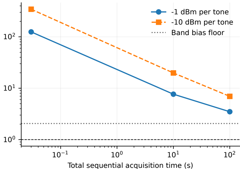
(b) 71 tones, 260–400 GHz
