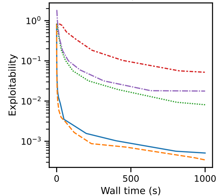
Goofspiel-6
