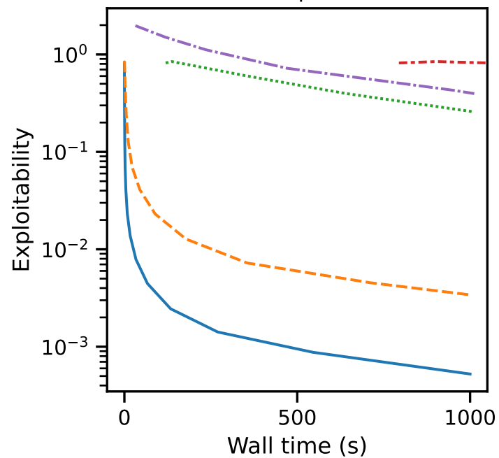
Goofspiel-7
