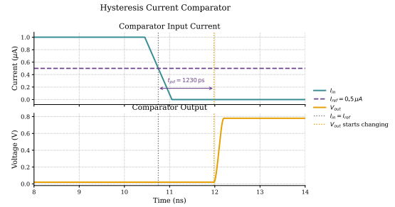
(d) Hysteresis
