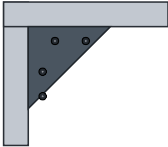
조인트 상세 A — 스틸 코너 거셋 (상·하단 4곳)
