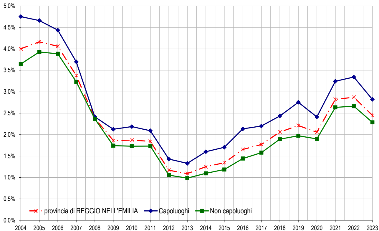
Figura 43: IMI per intera provincia, capoluogo e comuni non capoluogo
