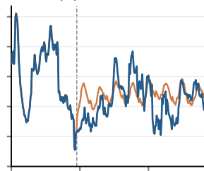
(d) TimeMixer
