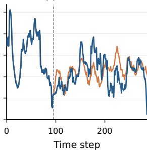
(f) PatchTST
