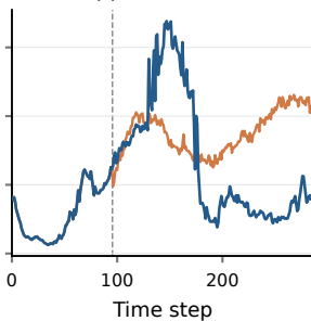
(f) PatchTST
