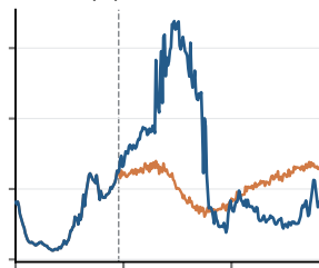
(d) TimeMixer
