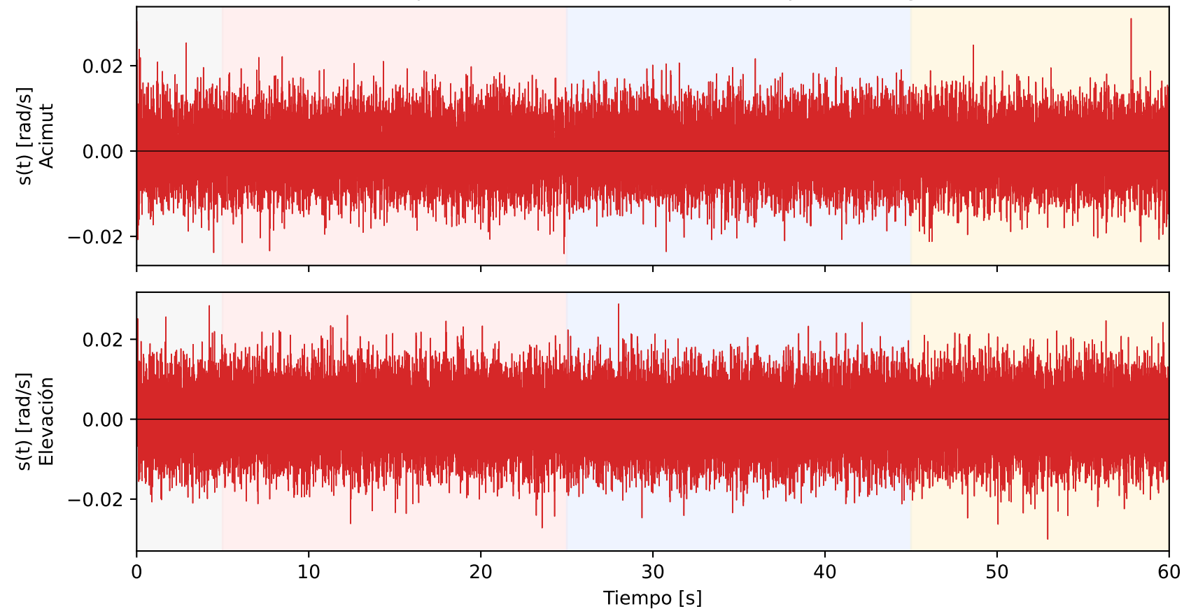
Superficie deslizante s(t) — SMC Super-Twisting
