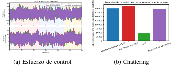
Fig. 4. (a) Par de control aplicado por eje (acimut, elevación) para las cuatro leyes de control. (b) Índice de chattering (variación total del par) por controlador.
