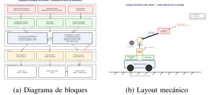
Fig. 5. (a) Diagrama de bloques del prototipo: perturbaciones controladas → sensorica → cómputo (MCU tiempo real + SBC) → actuación → planta física, con realimentación óptica de validación. (b) Layout mecánico del robot (vista lateral, no a escala): base móvil, actuadores de acimut/elevación, tubo óptico simulado con contrapeso y carga útil láser+PSD.
