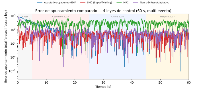
Fig. 2. Error de apuntamiento total comparado (escala logarítmica) para las cuatro leyes de control, bajo perturbación multi-evento idéntica.
