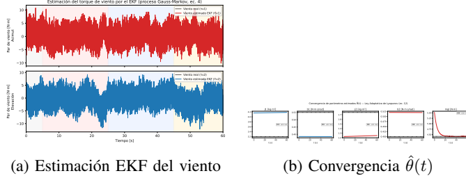
Fig. 3. (a) Estimación del torque de viento (proceso Gauss-Markov) por el EKF, comparada con el valor real, para acimut y elevación. (b) Convergencia de los parámetros estimados \hat{\theta}(t) hacia sus valores reales (líneas punteadas), ley Adaptativa-Lyapunov.
