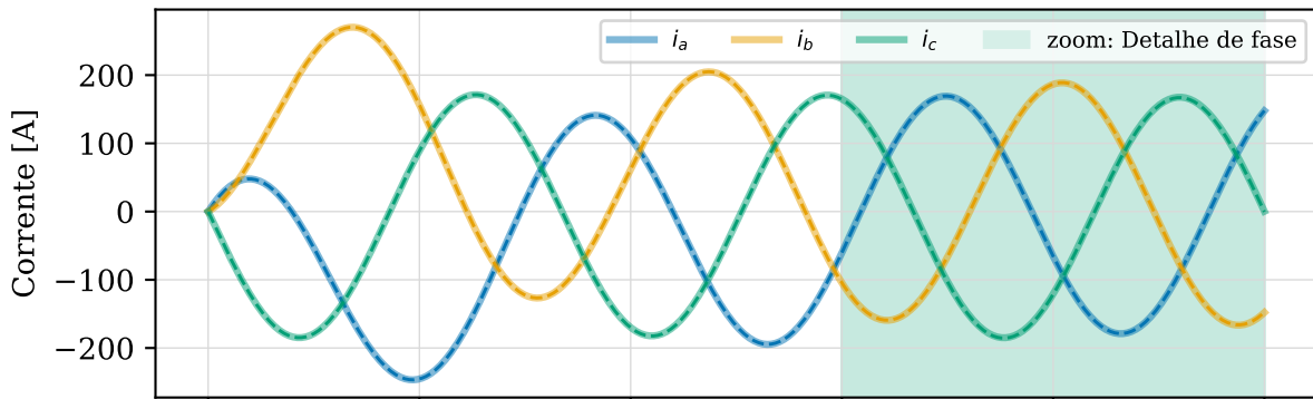
L2 — Partida senoidal 60 Hz: correntes (— VHDL, - - C)
