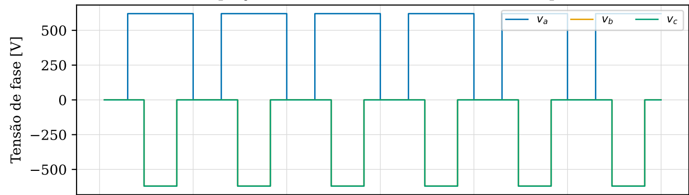
L3 — PWM replay — Seno 6 ms: estímulo PWM → resposta, 0-6 ms
