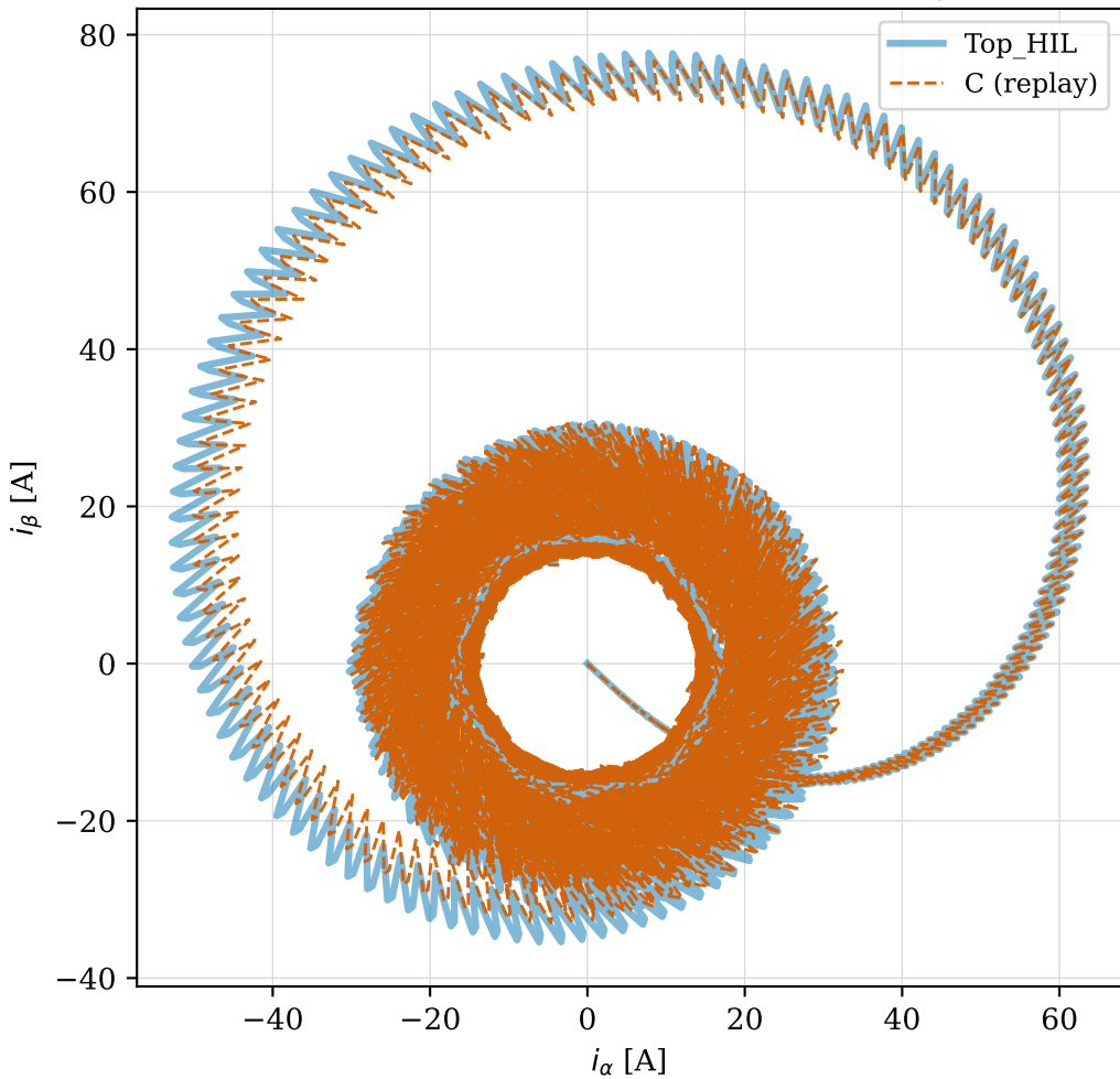
L3 — PWM replay — V/f 2 s: trajetória i_\beta \times i_\alpha
