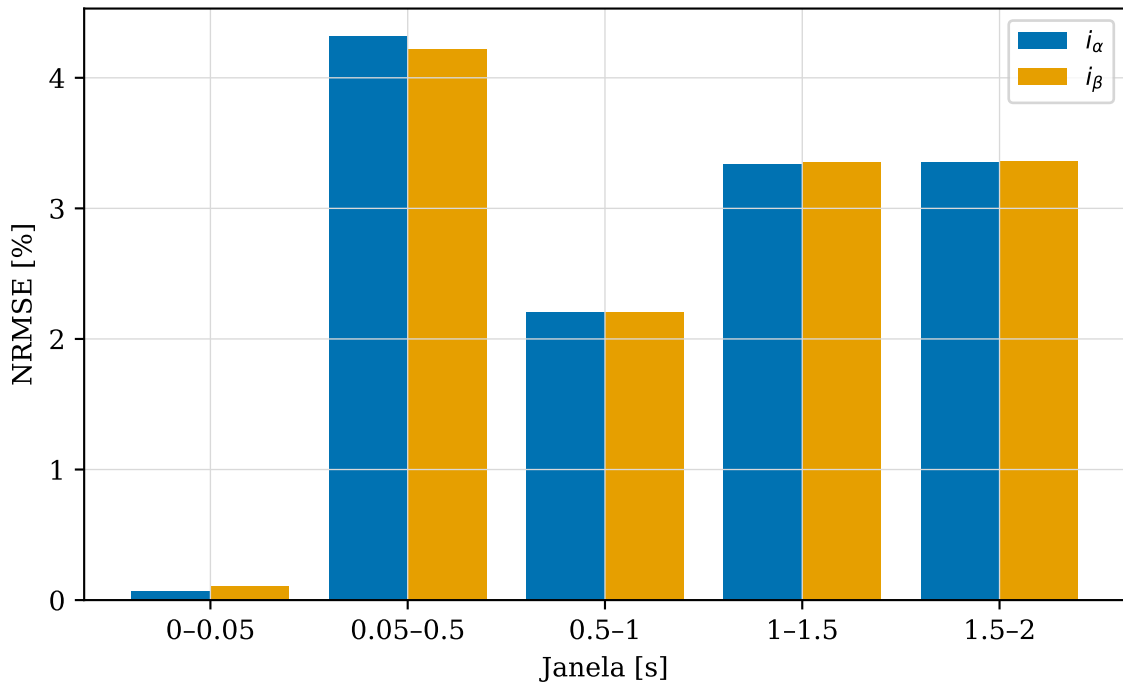
L3 — PWM replay — V/f 2 s: NRMSE por janela
