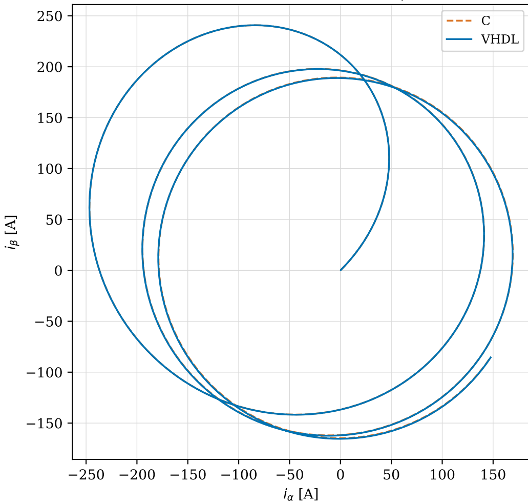
L2 — Seno 60 Hz: trajetória i_\beta \times i_\alpha
