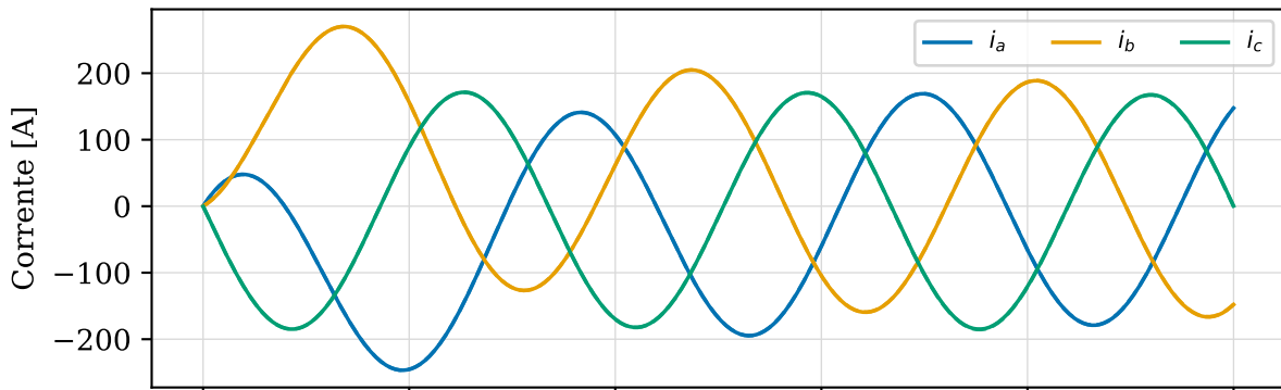
L2 — Seno 60 Hz: correntes (— VHDL, - - C)
