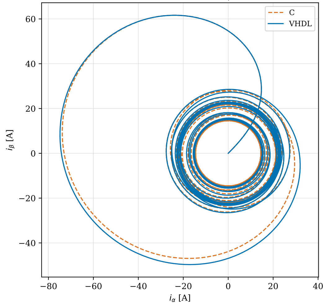
L2 — V/f 2 s: trajetória i_\beta \times i_\alpha
