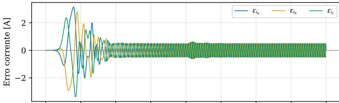
L2 — V/f 2 s: erro VHDL — C
