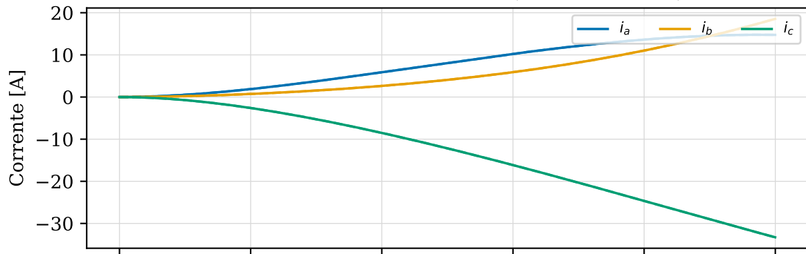
L2 — V/f 50 ms: correntes (— VHDL, - - C)
