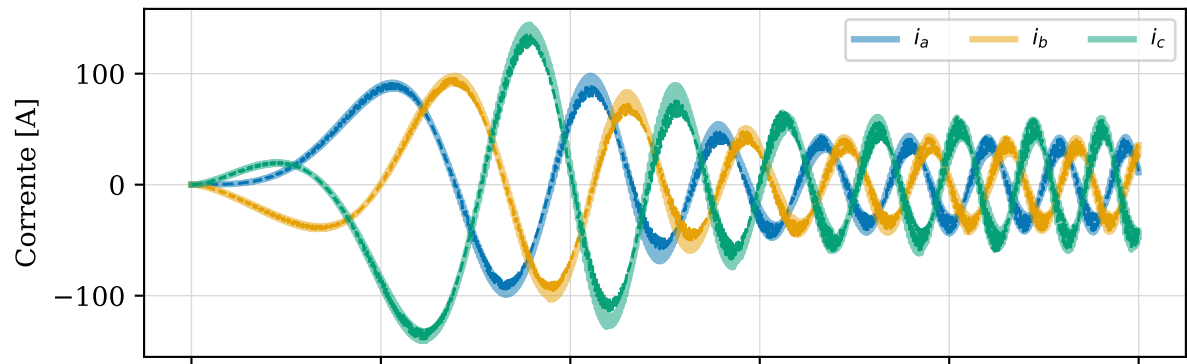
L4 — A3 — t_{acc}=1 s, carga leve · Partida: correntes (— FPGA (real), - - Modelo C)
