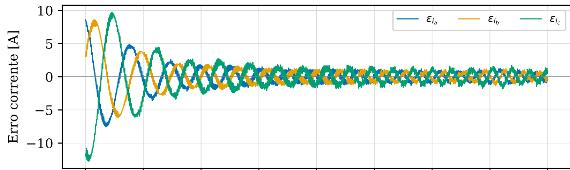
L4 — B1 — degrau 0,25→0,75 T_n · Partida: erro FPGA (real) — Modelo C
