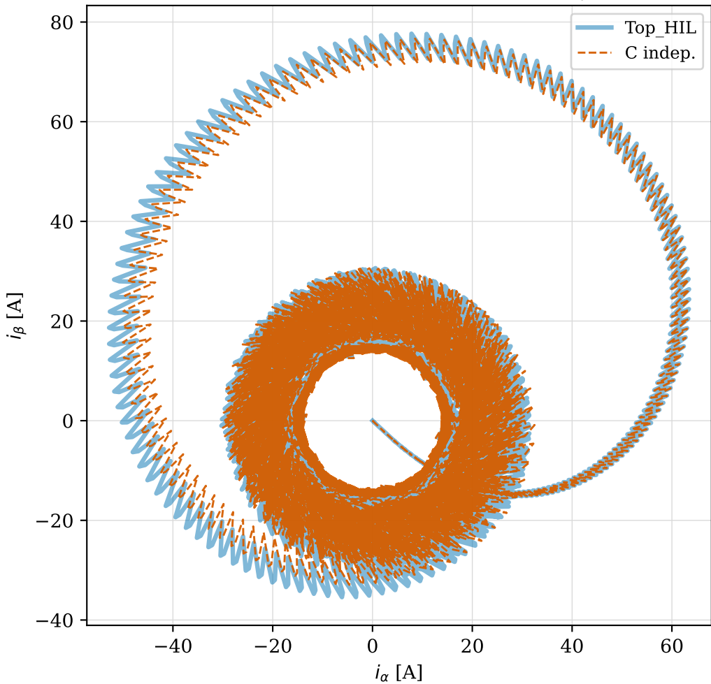
L3 — Full-stack — V/f 2 s: trajetória i_\beta \times i_\alpha
