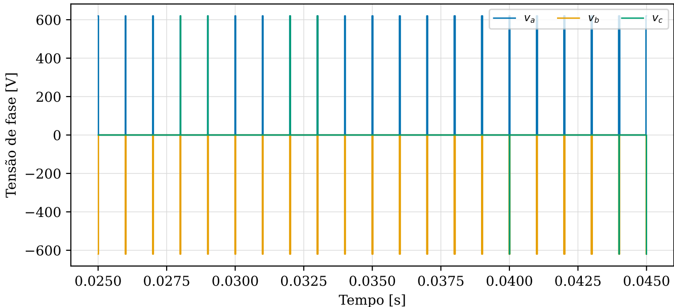
L3 — Full-stack — V/f 50 ms: estímulo PWM (saída NPC), 25–45 ms
