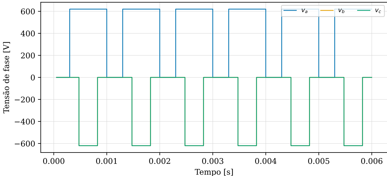
L3 — PWM replay — Seno 6 ms: estímulo PWM (saída NPC), 0-6 ms
