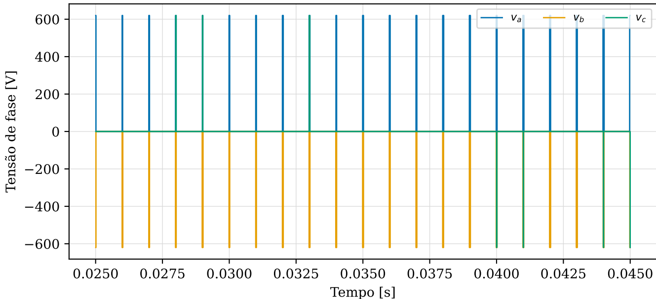
L3 — PWM replay — V/f 50 ms: estímulo PWM (saída NPC), 25-45 ms
