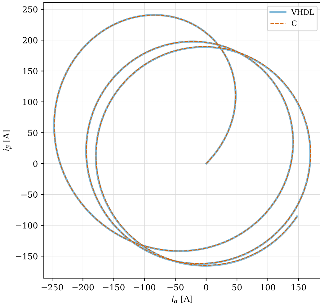
L2 — Partida senoidal 60 Hz: trajetória i_\beta \times i_\alpha
