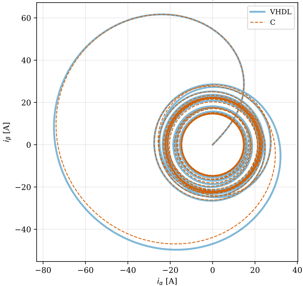
L2 — V/f 2 s: trajetória i_\beta \times i_\alpha
