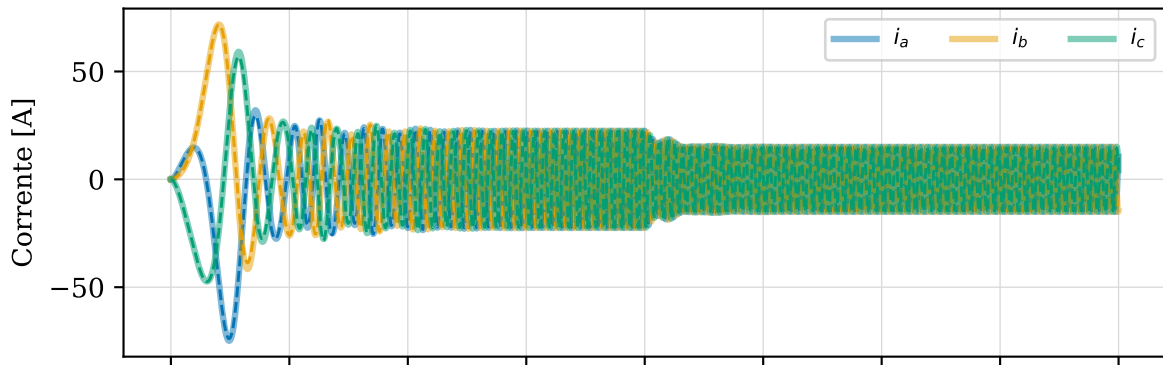
L2 — V/f 2 s: correntes (— VHDL, - - C)
