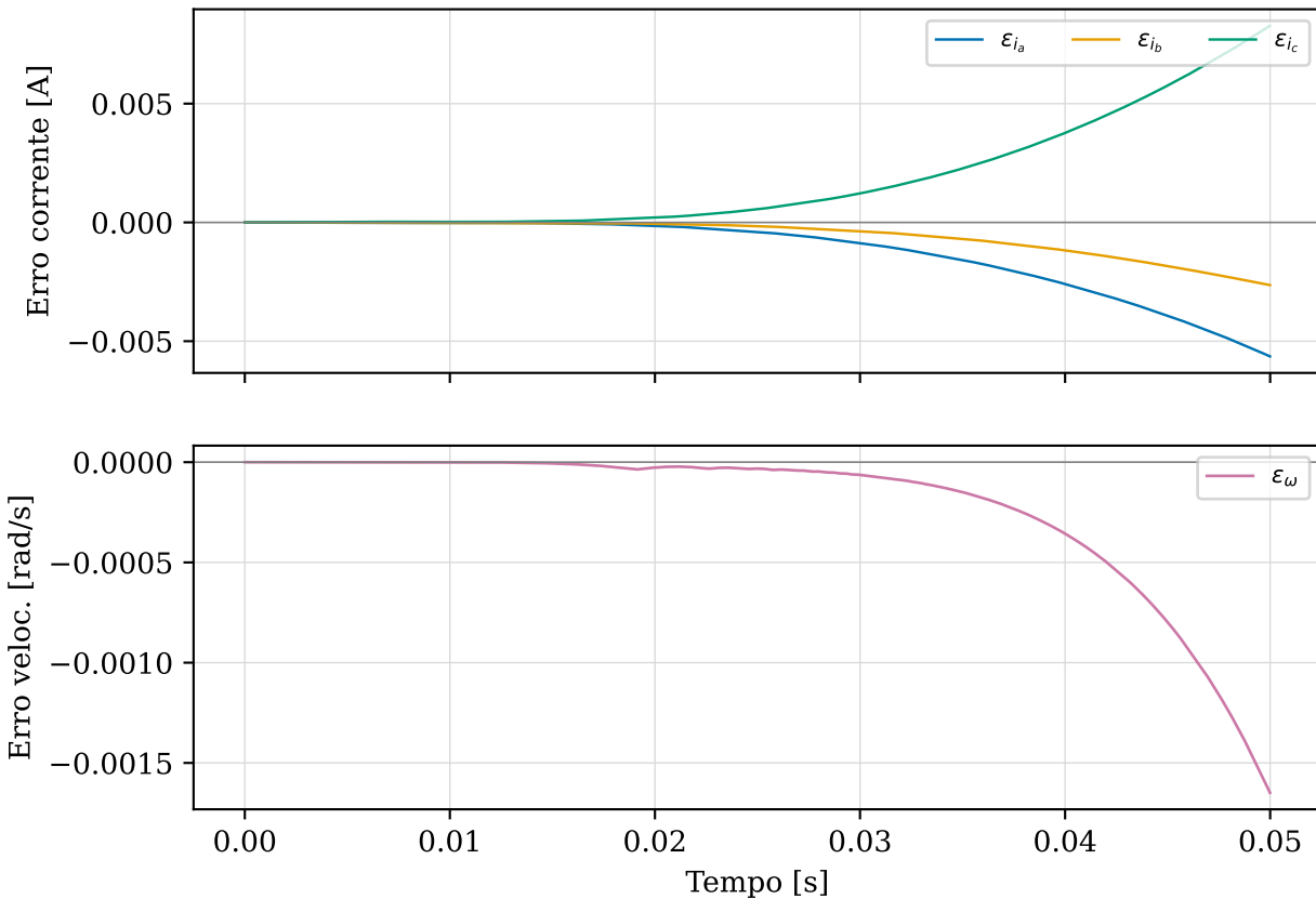
L2 — V/f 50 ms: erro VHDL — C
