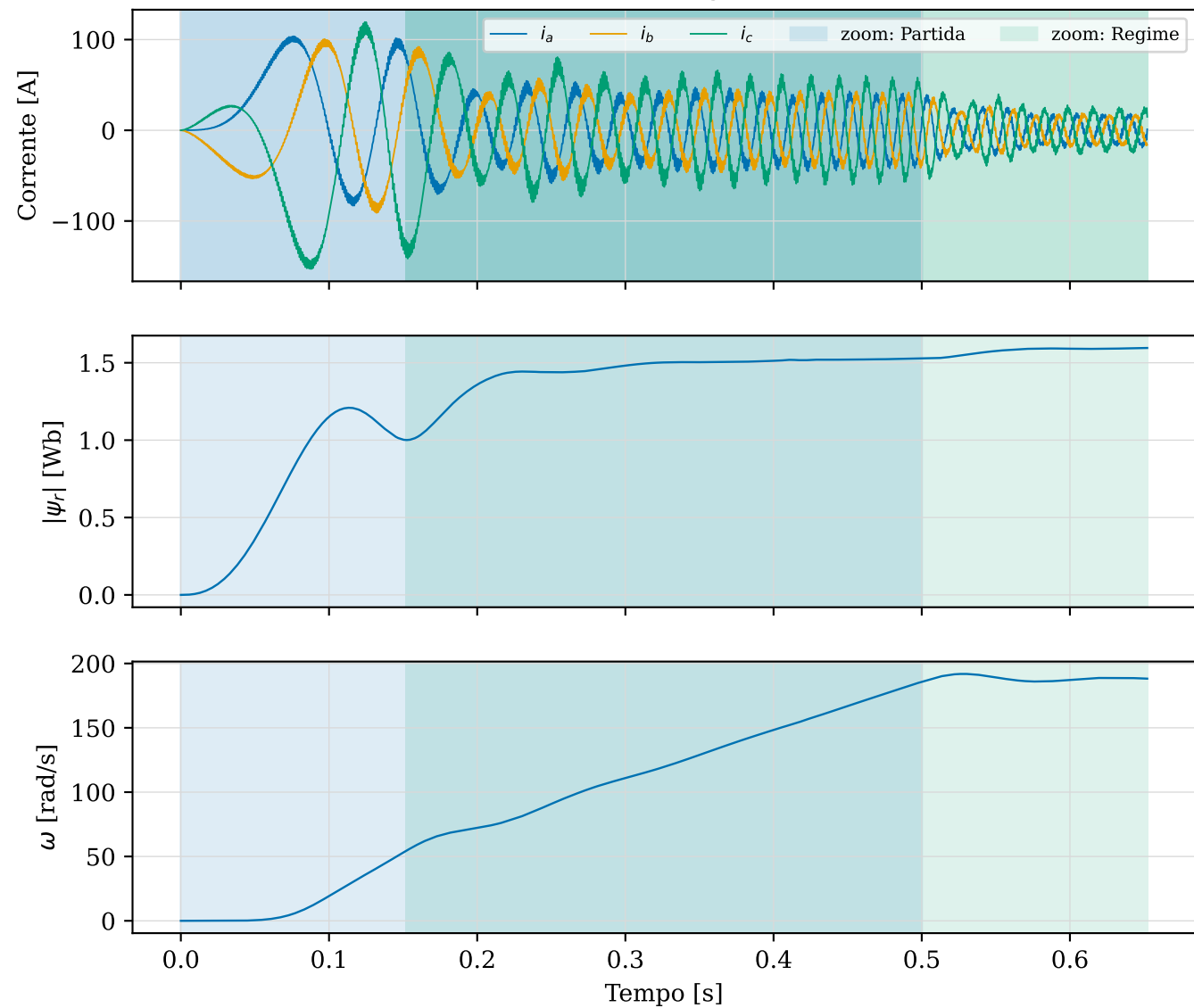
L4 — A1 — t_{acc}=0,5 s, vazio: visão geral da captura (FPGA real)
