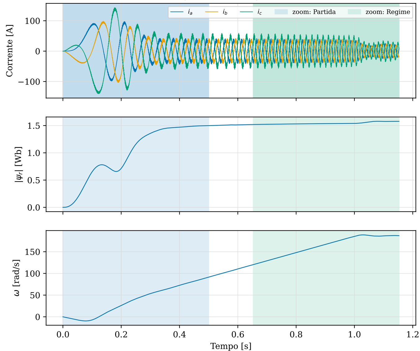
L4 — A3 — t_{acc}=1 s, carga leve: visão geral da captura (FPGA real)
