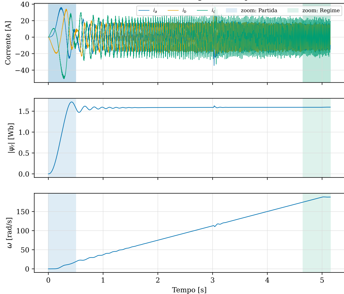
L4 — A5 — t_{acc}=5 s, vazio: visão geral da captura (FPGA real)
