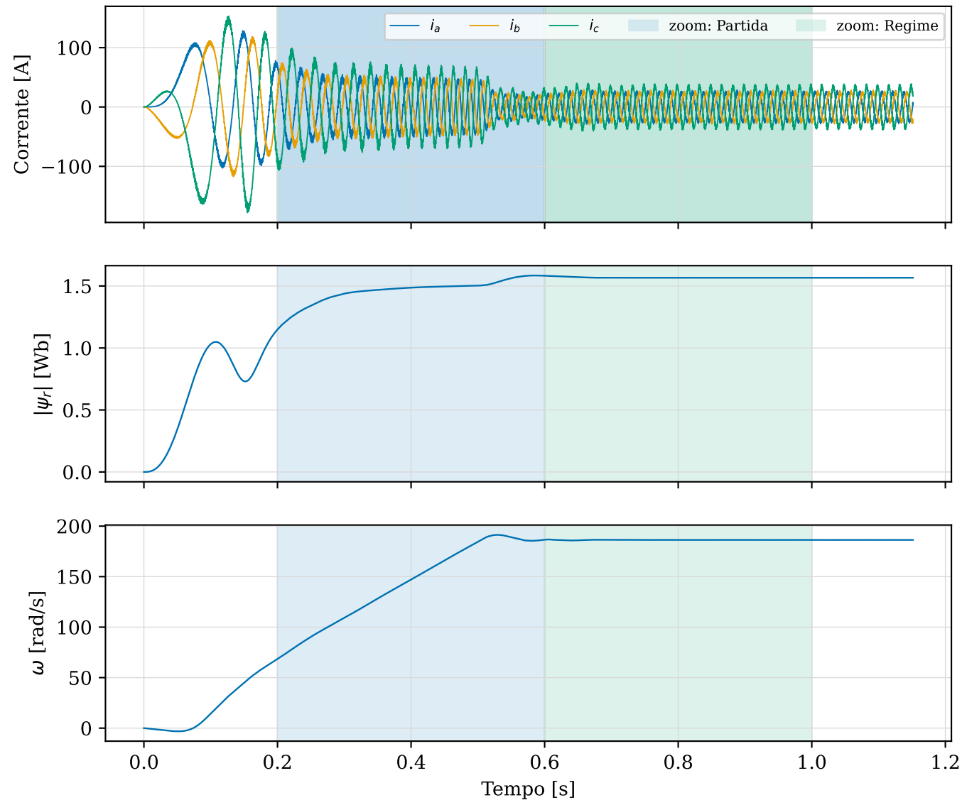
L4 — B1 — degrau 0,25→0,75 T n : visão geral da captura (FPGA real)
